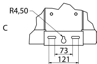
Orificios oblongos para fijación a la pared con tacos y tornillos Ø8
